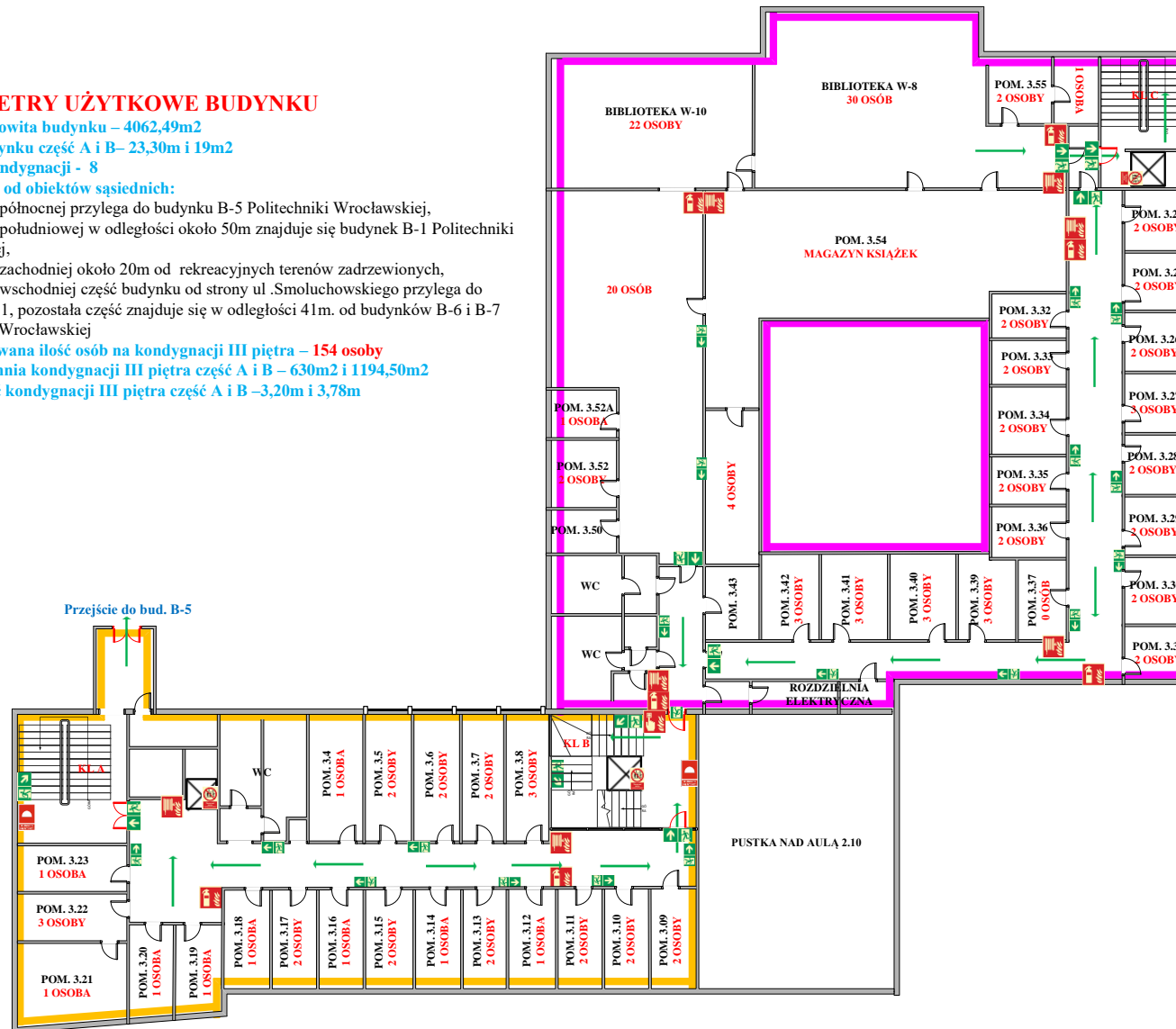
Rozmieszczenie urządzeń przeciwpożarowych oraz kierunków ewakuacji W BUDYNKU B-4 POLITECHNIKI WROCŁAWSKIEJ III PIĘTRO
