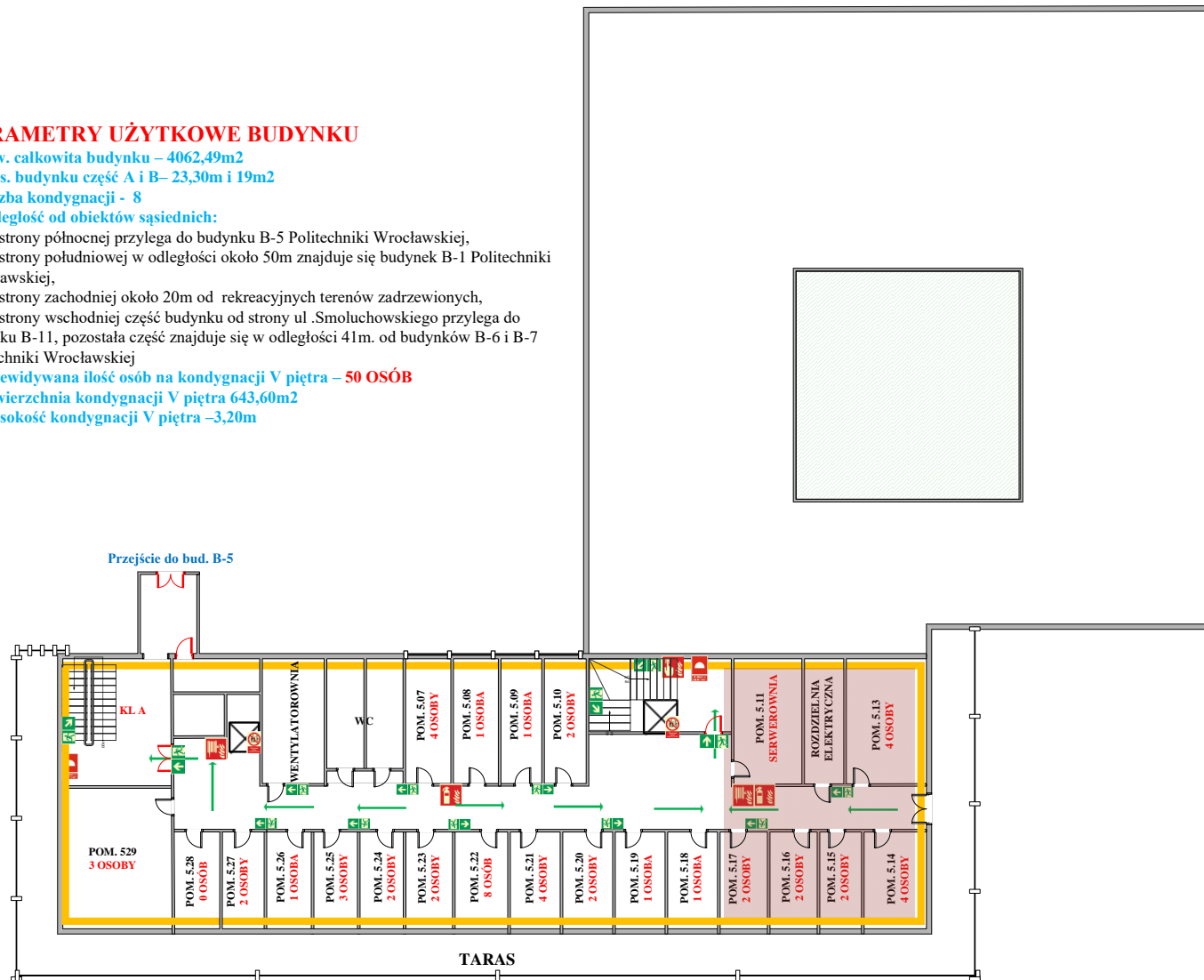
Rozmieszczenie urządzeń przeciwpożarowych oraz kierunków ewakuacji W BUDYNKU B-4 POLITECHNIKI WROCŁAWSKIEJ V PIĘTRO
