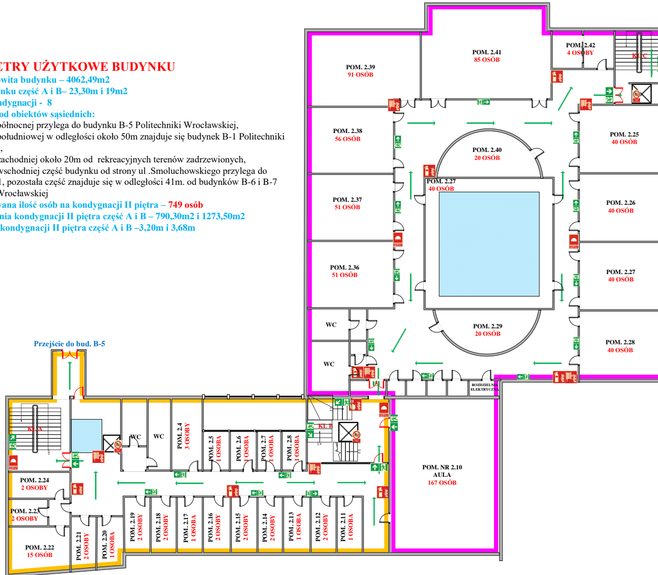
Rozmieszczenie urządzeń przeciwpożarowych oraz kierunków ewakuacji W BUDYNKU B-4 POLITECHNIKI WROCŁAWSKIEJ II PIĘTRO
