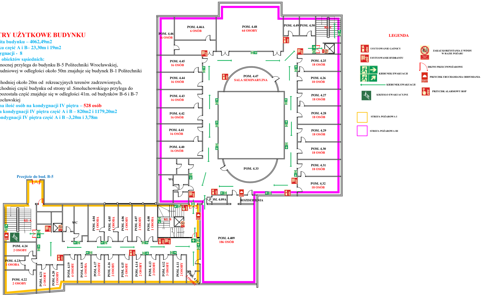
Rozmieszczenie urządzeń przeciwpożarowych oraz kierunków ewakuacji W BUDYNKU B-4 POLITECHNIKI WROCŁAWSKIEJ IV PIĘTRO
