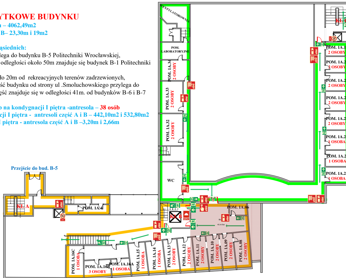
Rozmieszczenie urządzeń przeciwpożarowych oraz kierunków ewakuacji W BUDYNKU B-4 POLITECHNIKI WROCŁAWSKIEJ I PIĘTRO ANTRESOLA
