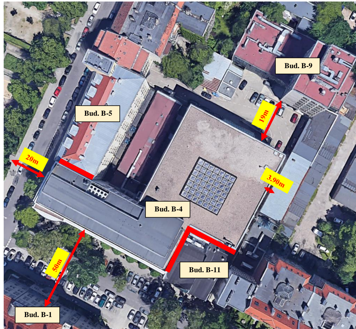
ODLEGŁOŚĆ BUDYNKU B-4 POLITECHNIKI WROCŁAWSKIEJ OD OBIEKTÓW SĄSIEDNICH
