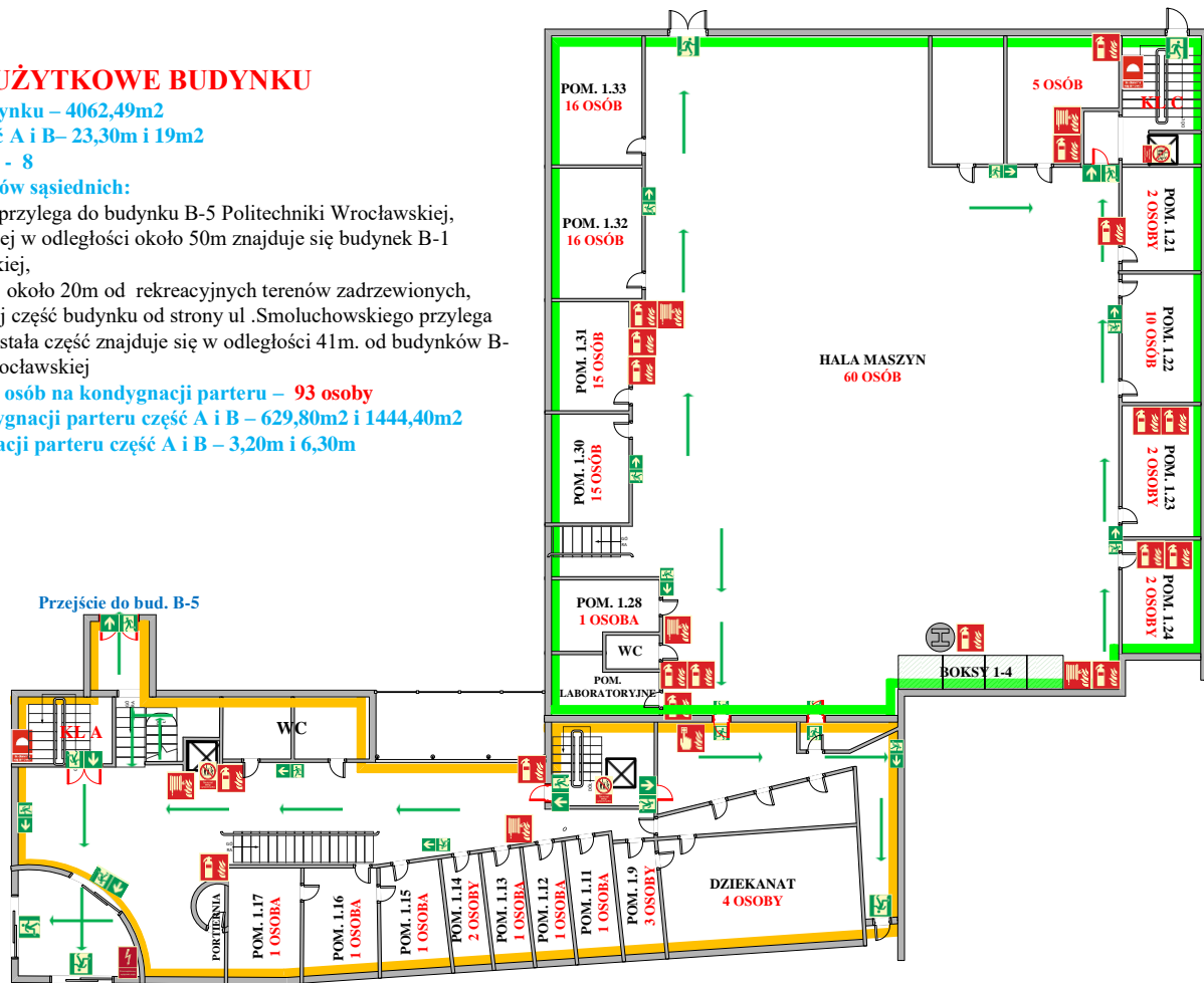
Rozmieszczenie urządzeń przeciwpożarowych oraz kierunków ewakuacji W BUDYNKU B-4 POLITECHNIKI WROCŁAWSKIEJ PARTER
