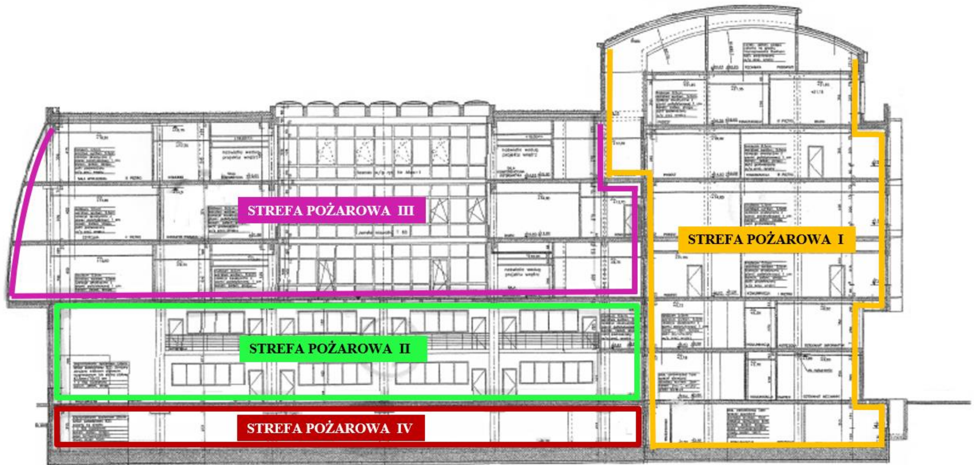
PRZEKRÓJ BUDYNKU B-4 POLITECHNIKI WROCŁAWSKIEJ Z OZNACZENIEM STREF POŻAROWYCH
